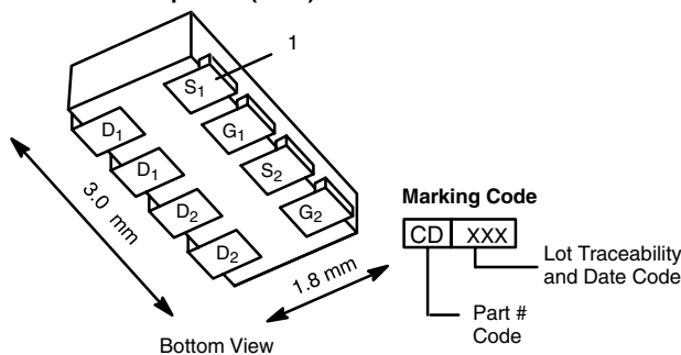
1206-8 ChipFET ® (Dual)
